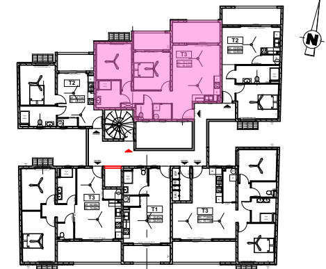
ETAGE 2
