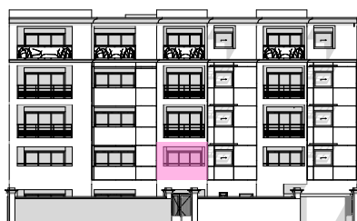
Façade Nord
